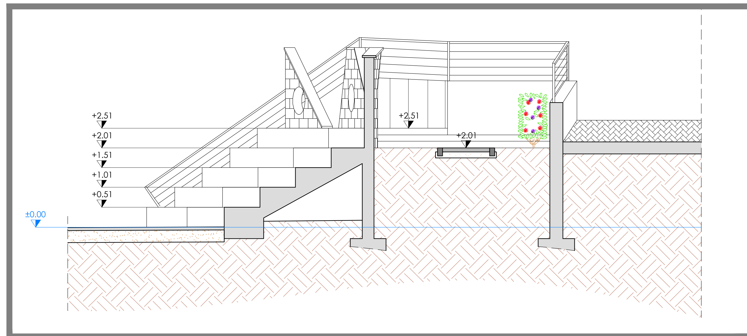
SEZIONE A-A
