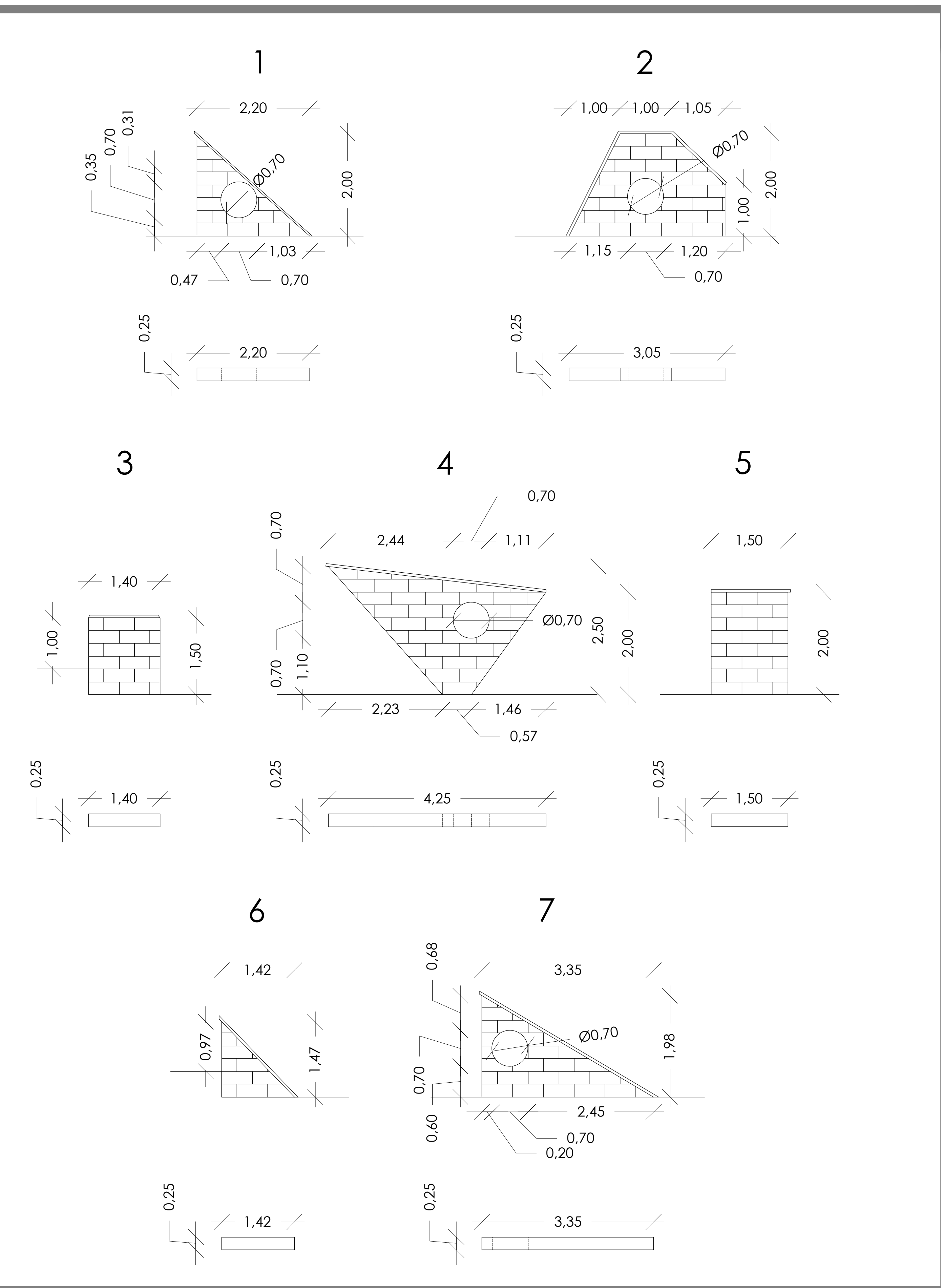
PARTICOLARI COSTRUTTIVI
