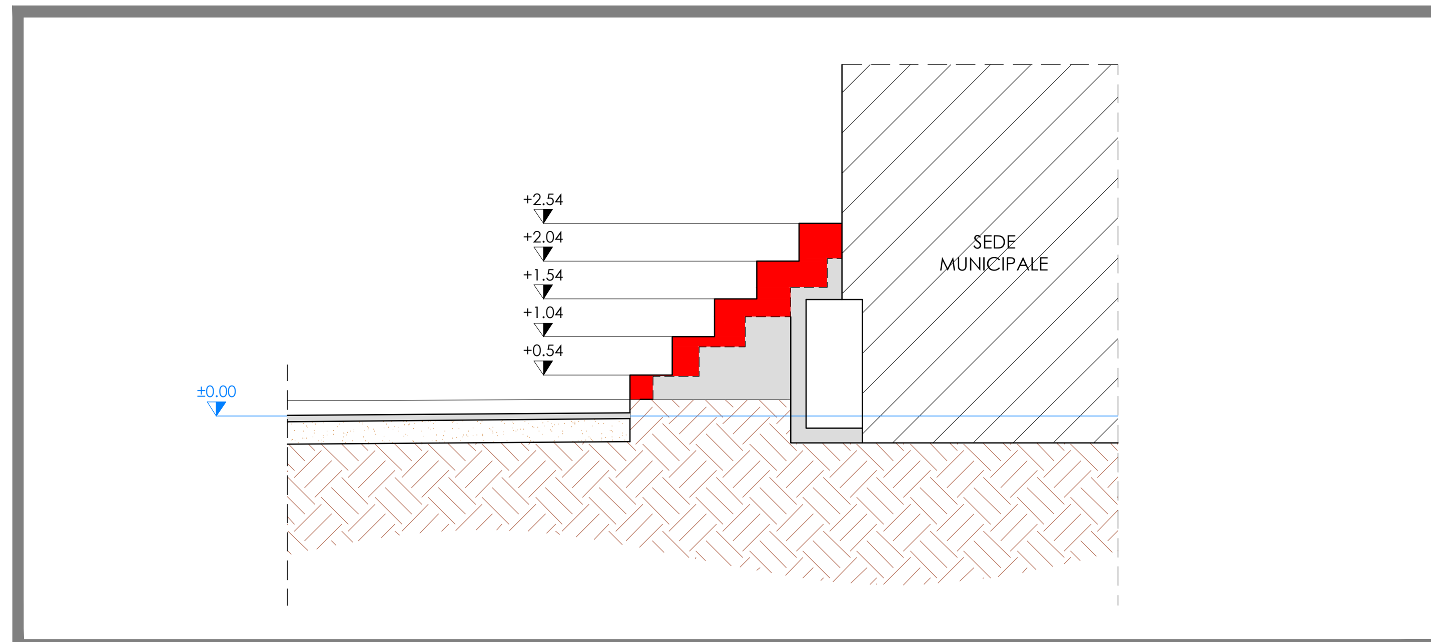
SEZIONE B-B
