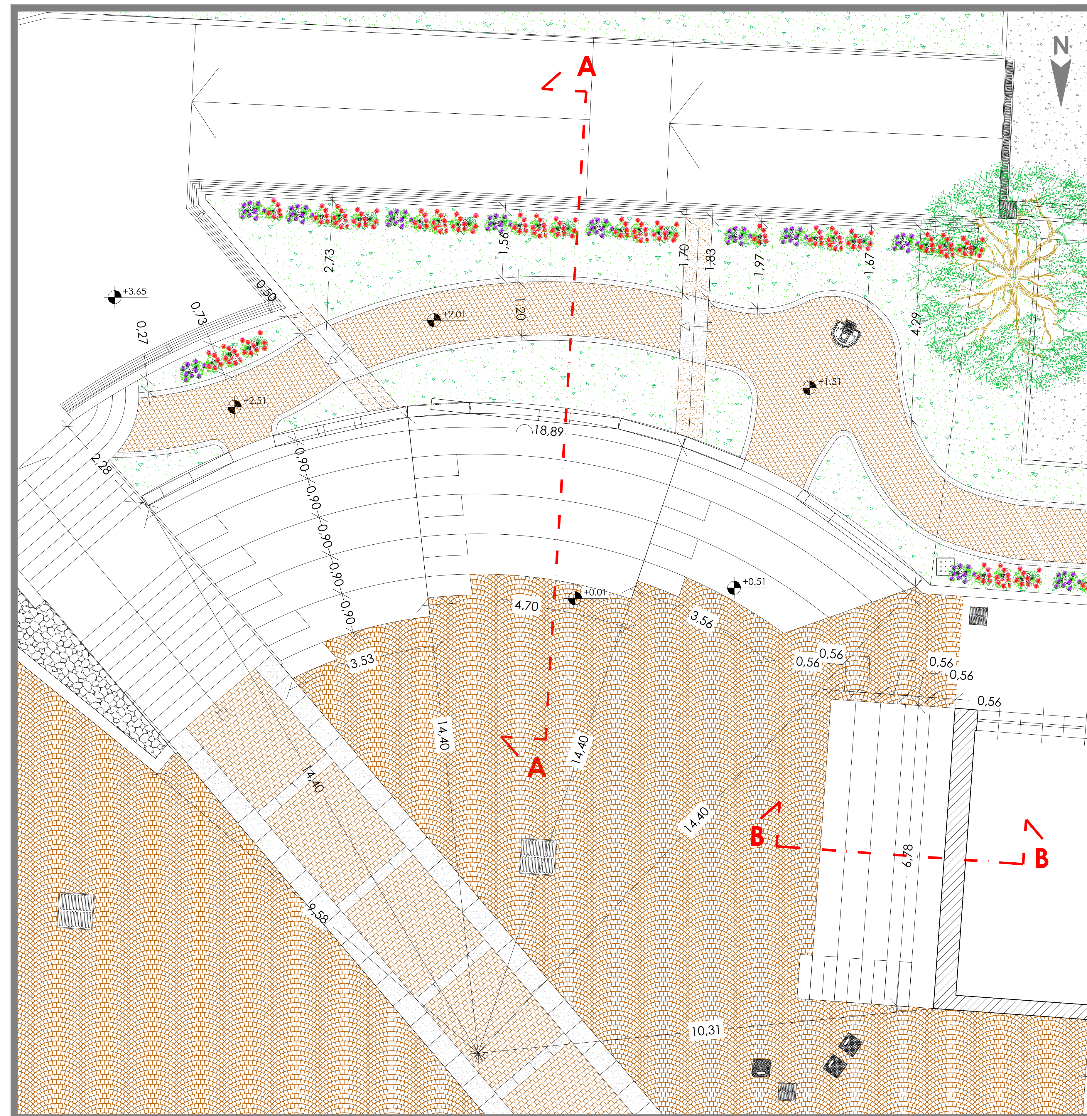
PLANIMETRIA
