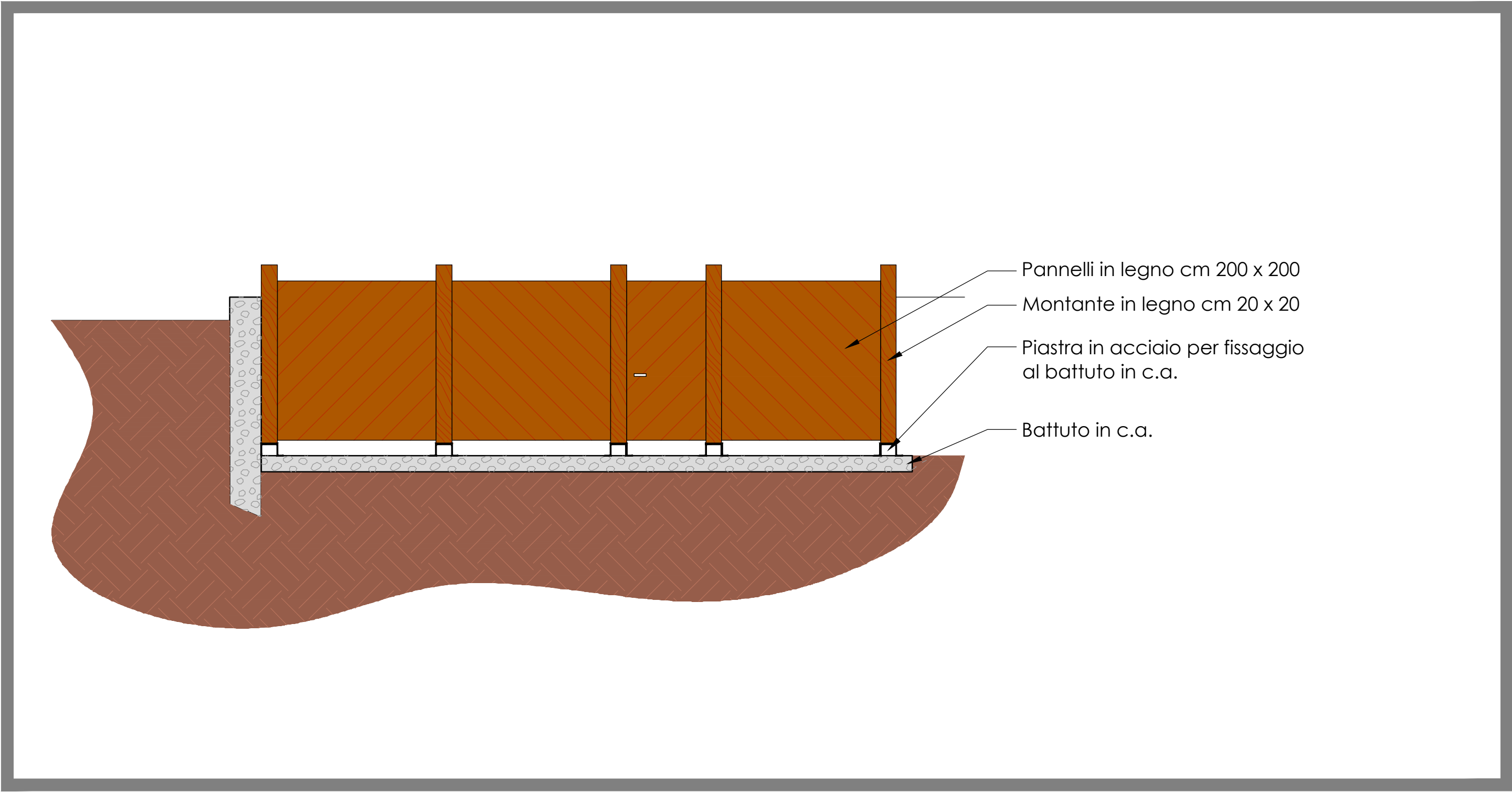
PROSPETTO
