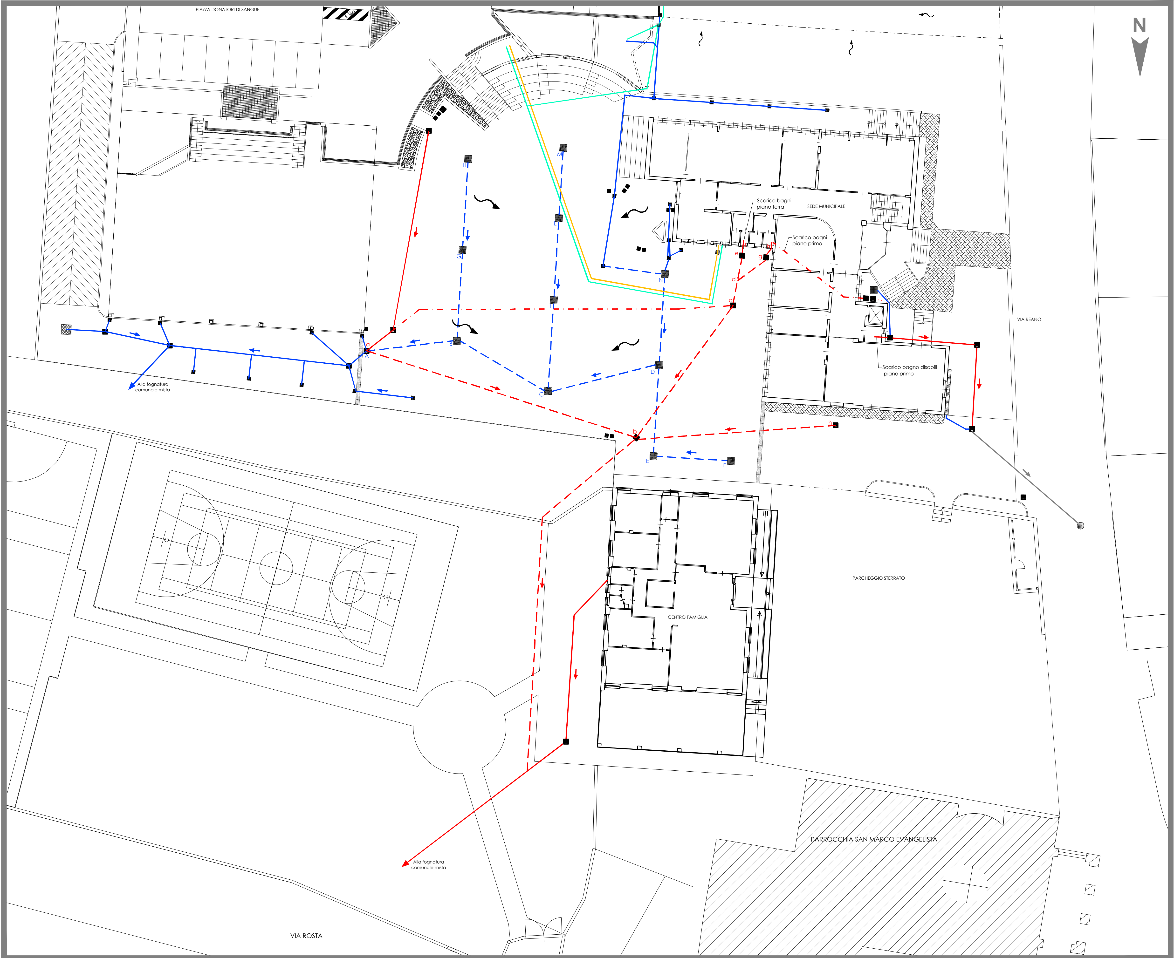
PLANIMETRIA GENERALE - RETI SERVIZI
